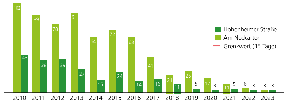
Abbildung 28: Feinstaubbelastung: \text{PM}_{10} > 50 \mu\text{g}/\text{m}^3 für zwei verkehrsnahen Messstellen (Angaben in Anzahl Tage)
