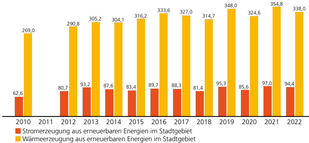
Abbildung 62: Wärme- bzw. Stromerzeugung aus erneuerbaren Energien im Stadtgebiet (Angaben in GWh)
