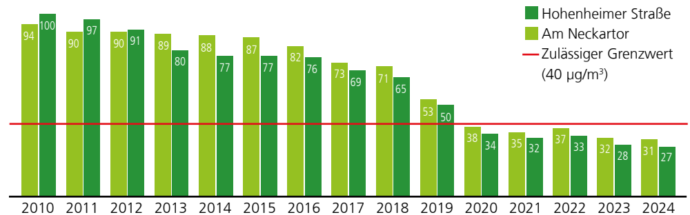
Abbildung 27: Stickstoffbelastung: Jahresmittelwerte \text{NO}_2 für zwei verkehrsnahen Messstellen (Angaben in \mu\text{g}/\text{m}^3 )
